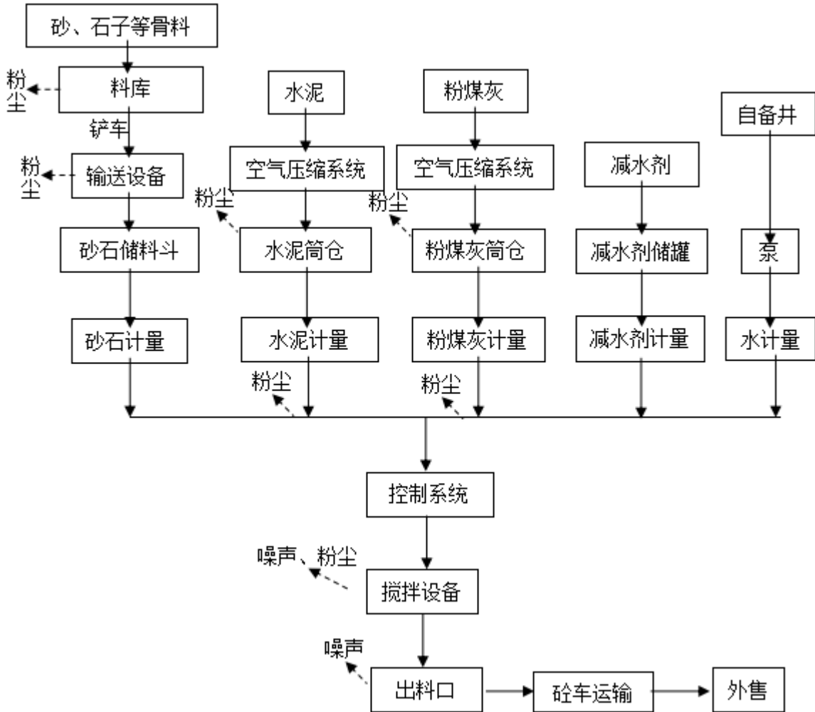
图3 产品工艺流程示意图
