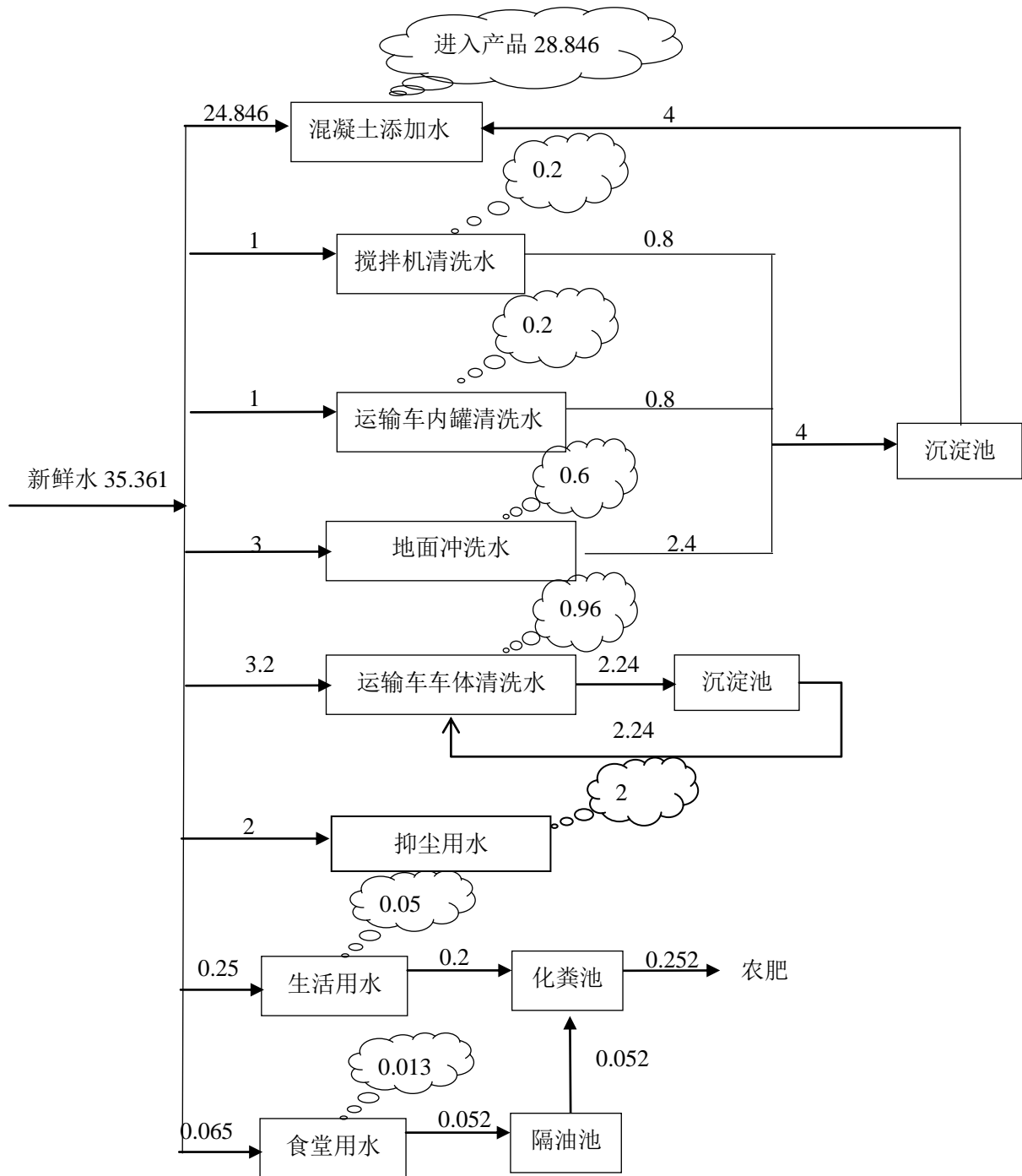
图 4 项目运营期水平衡图 (单位: m^3/d )
